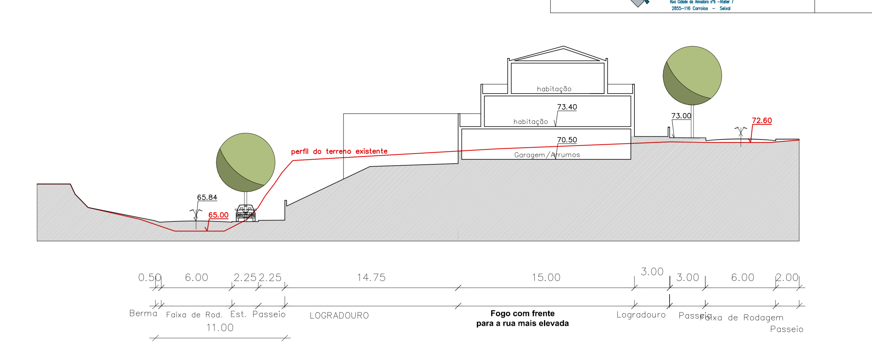
PERFIL A9
