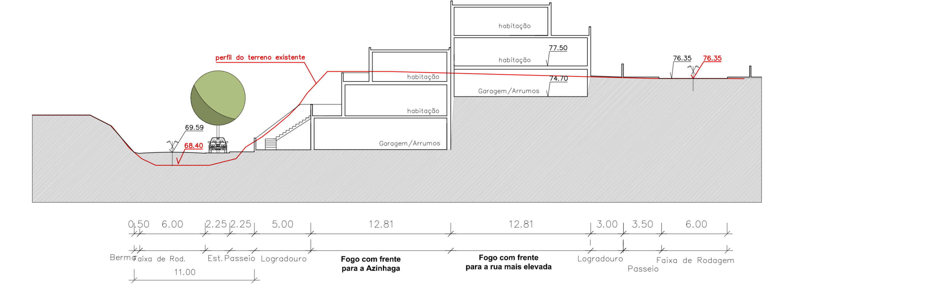
PERFIL A7
