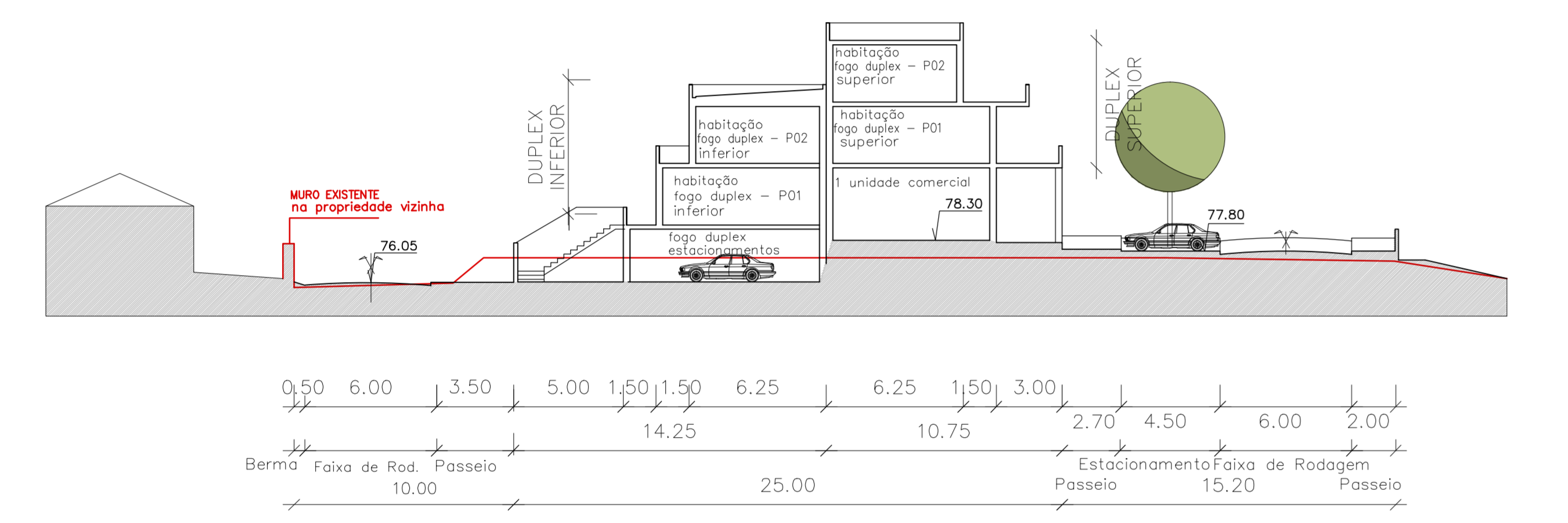
PERFIL A2
