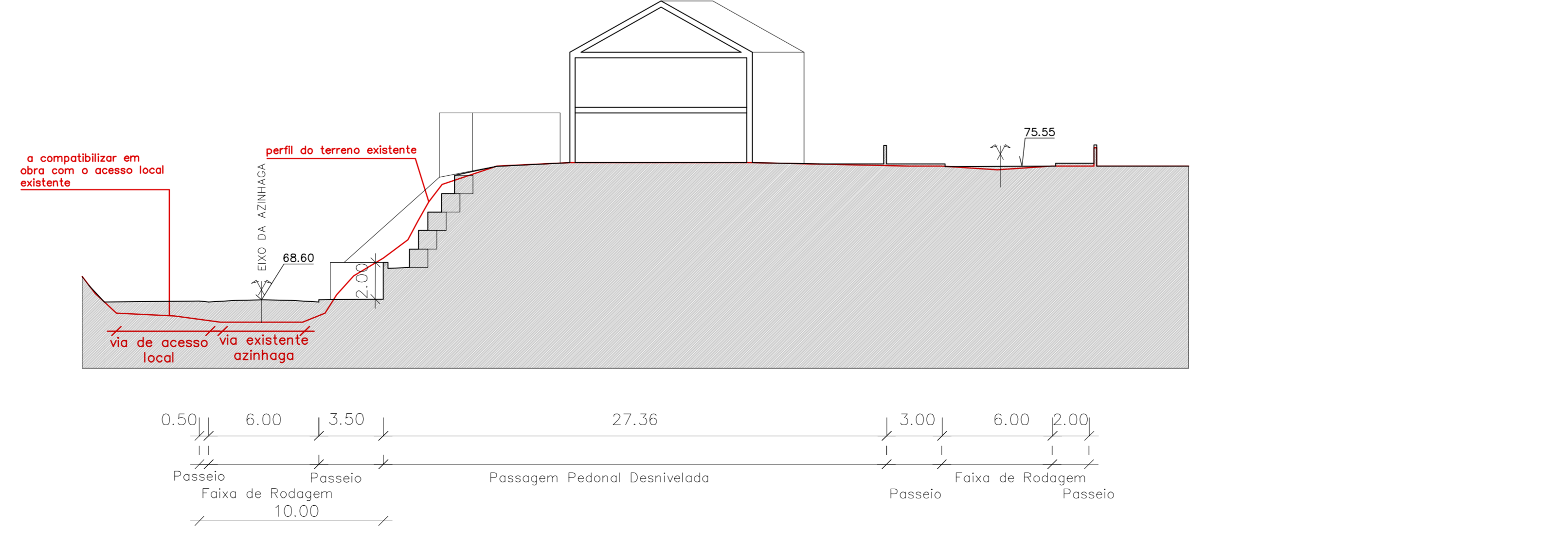
PERFIL A8
