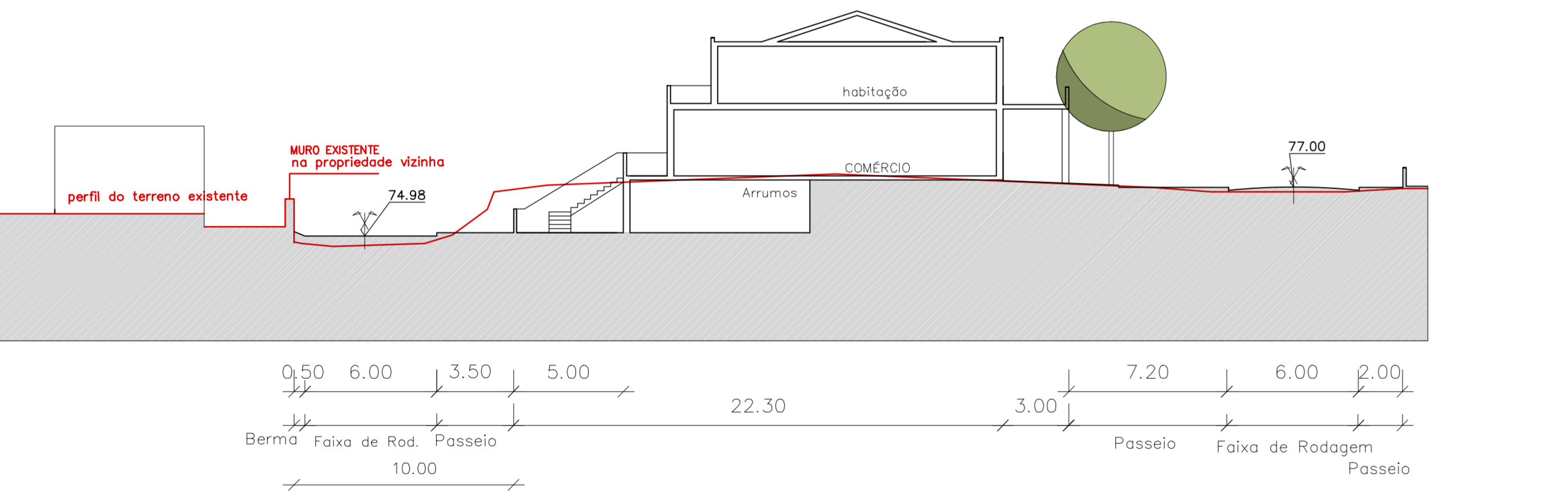
PERFIL A3
