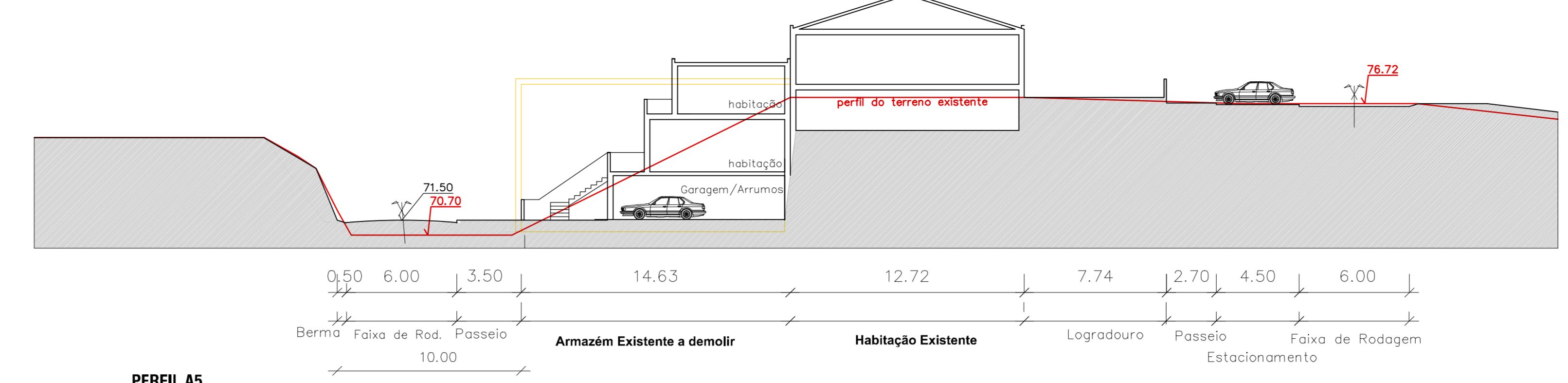
PERFIL A5
