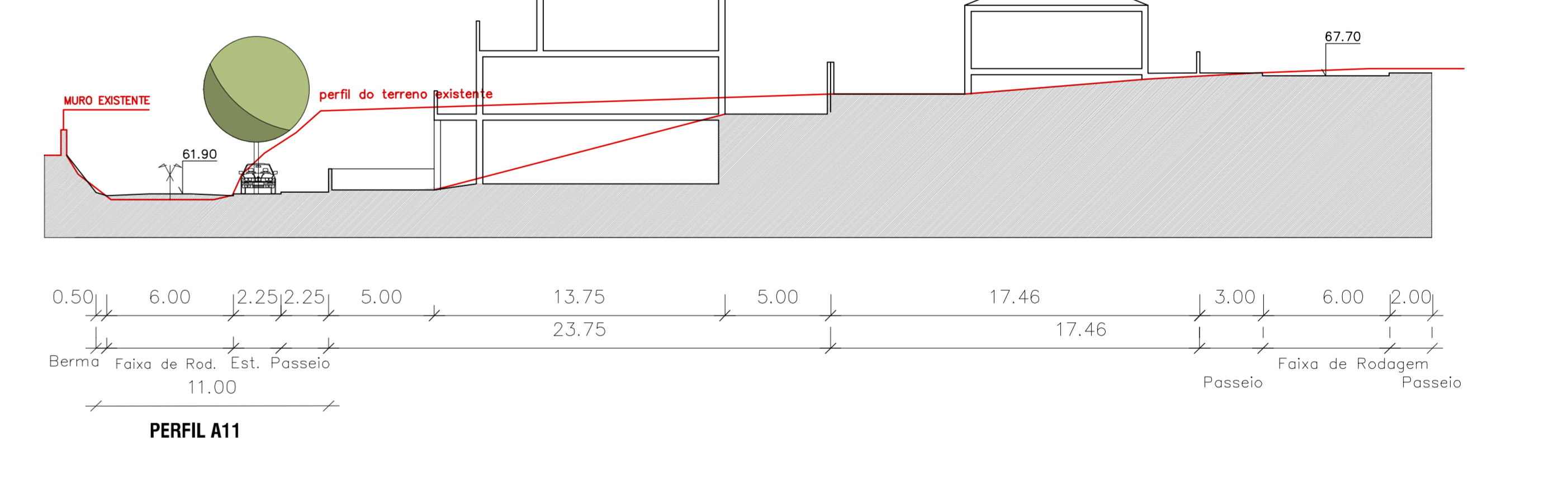
PERFIL A11
