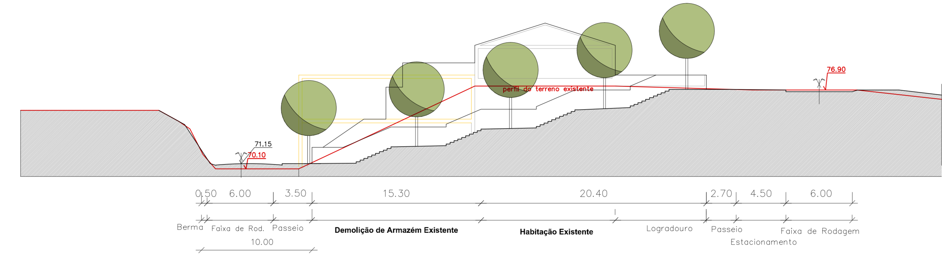
PERFIL A6
