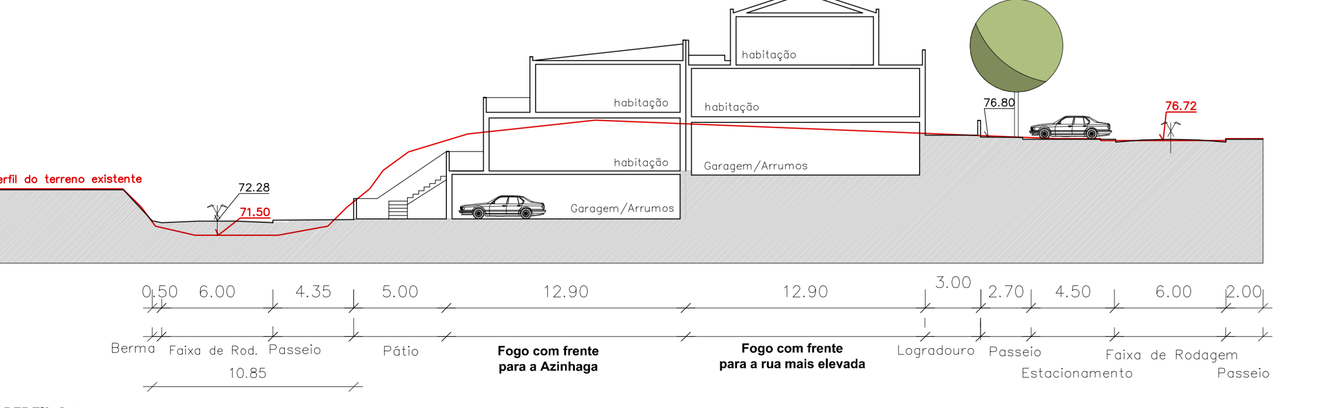
PERFIL A4
