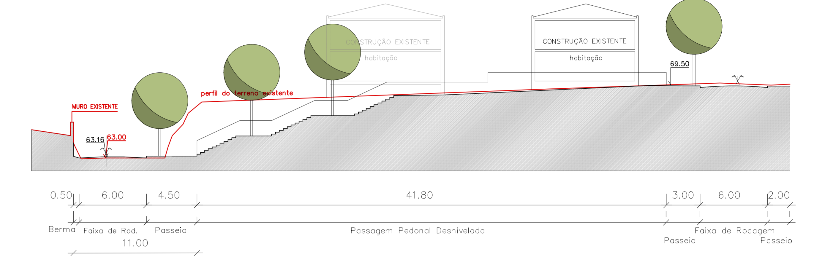
PERFIL A10
